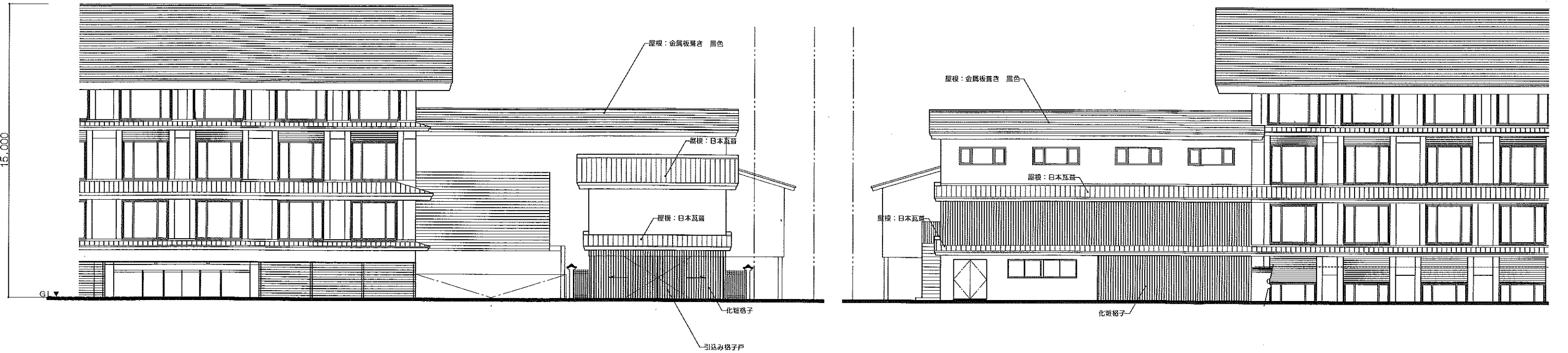
東側立面図(西洞院通)
