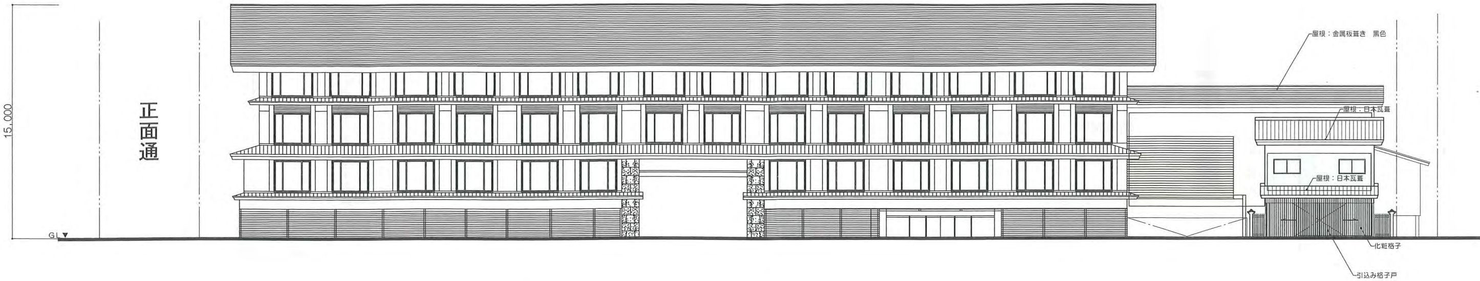
東側立面図(西洞院通)
